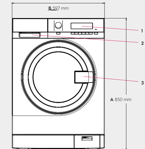
Frontal
