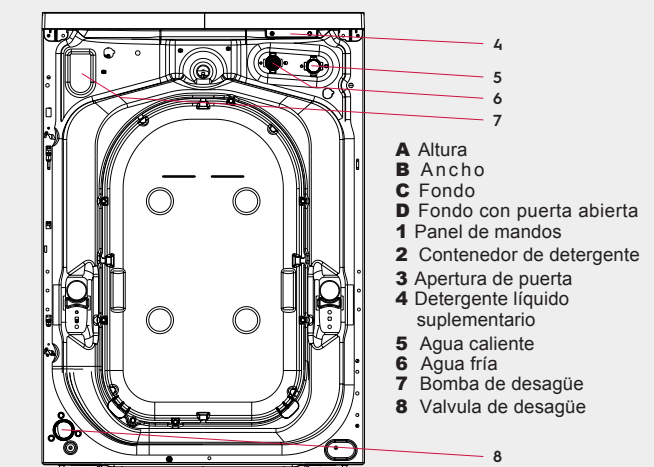
Parte trasera
